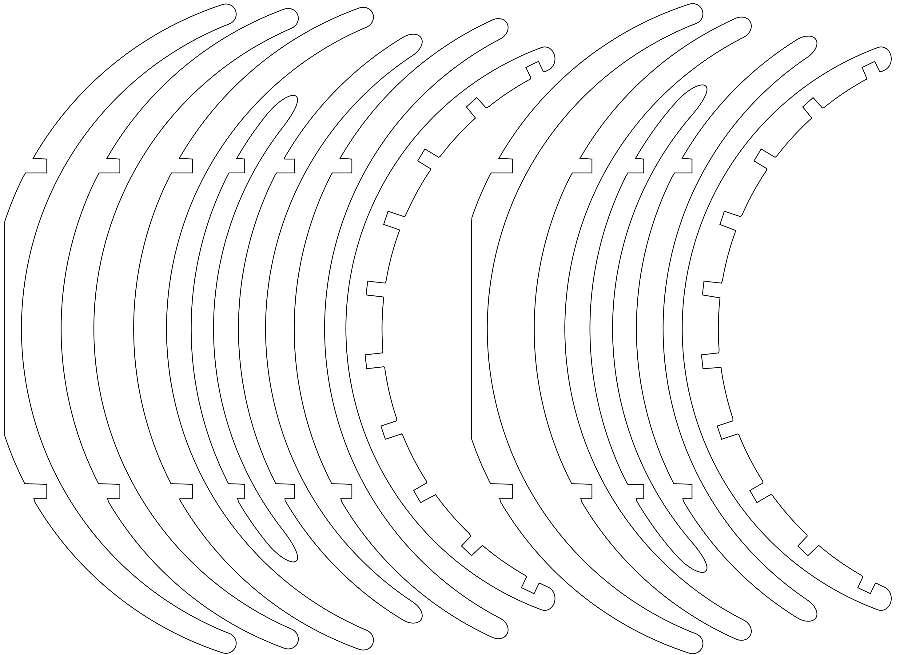
Fruitbowl „Sphere“ - ZenziWerken - 6.5 mm Plywood
